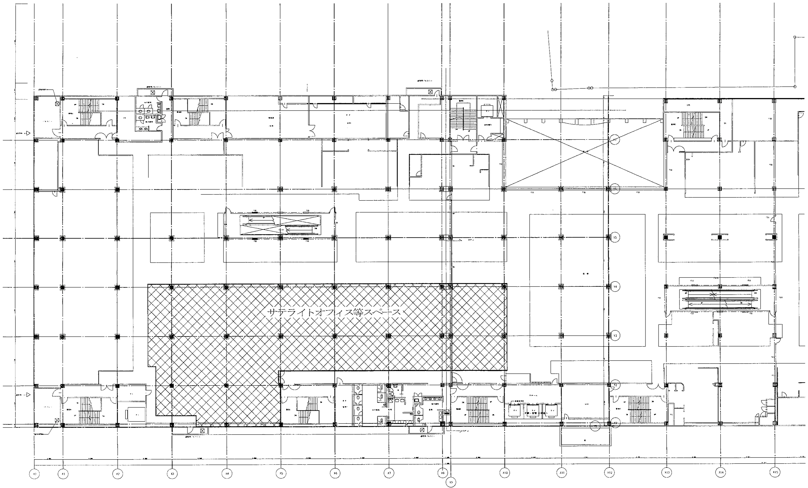
アルネ津山3階平面図 A3 1/300
